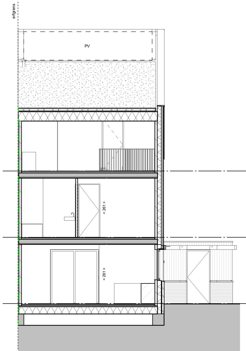
dwarsdoorsnede
