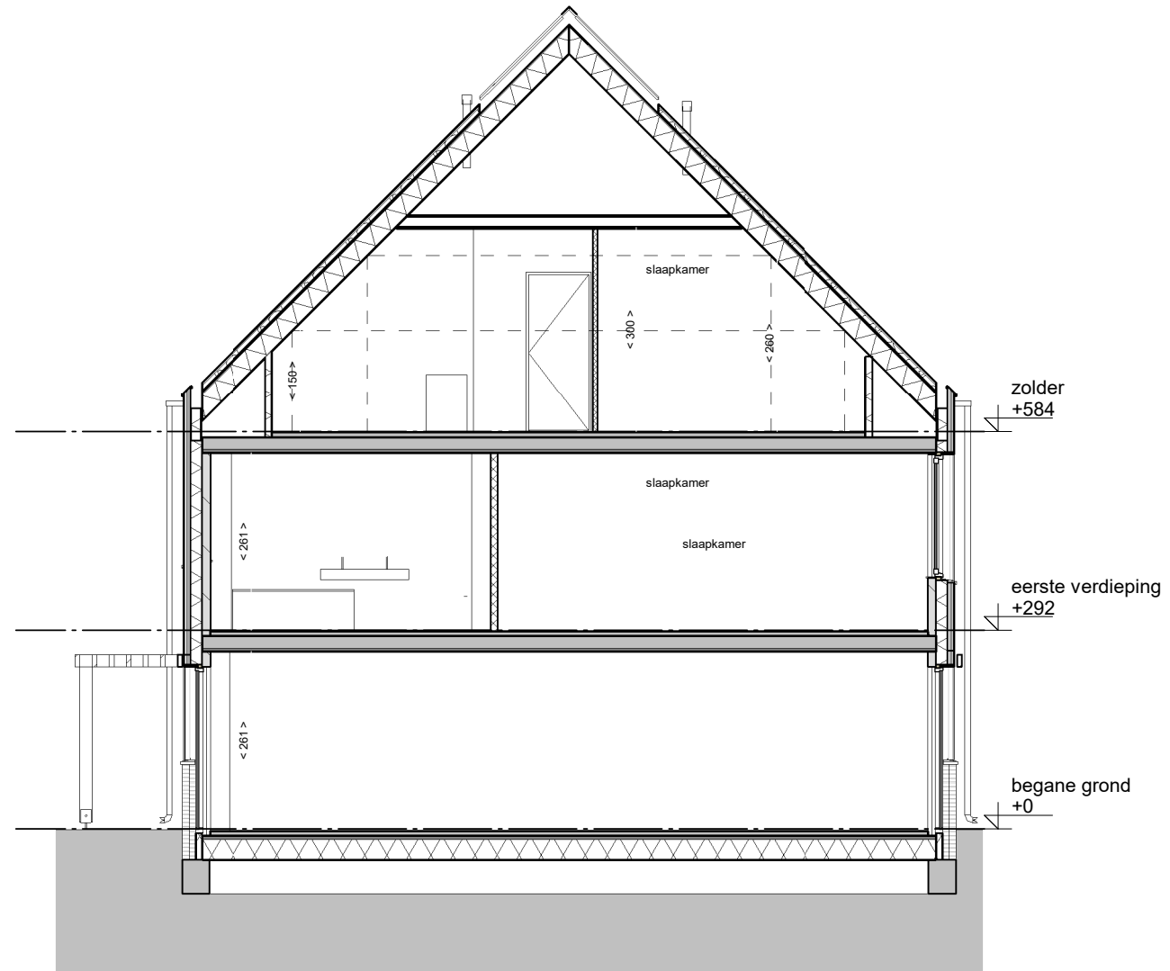
langsdoorsnede
